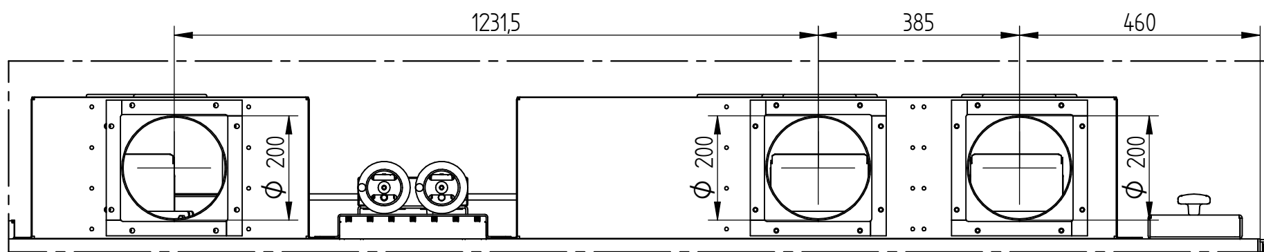
RÉSZLET A
